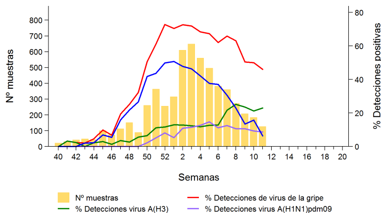
Figura 4. Muestras centinela analizadas y porcentaje de detecciones de virus de la gripe. Temporada 2017-18. España
