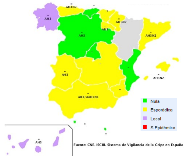
Figura 4. Nivel de difusión de la gripe. Semana 13/2019. Temporada 2018-19. España
