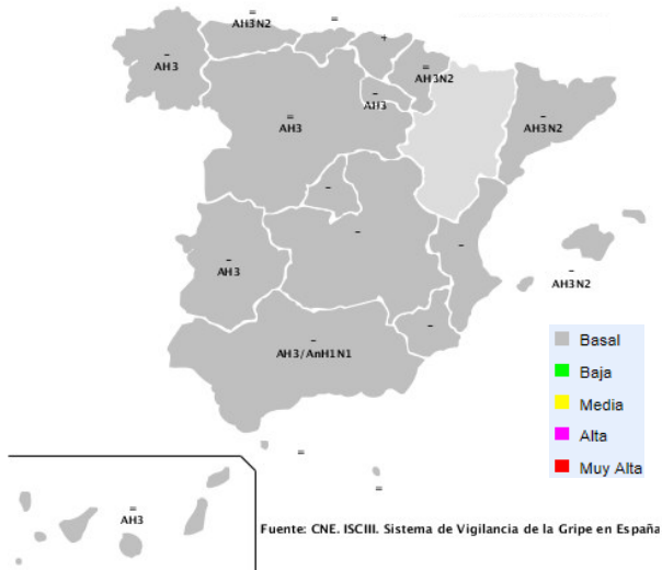
Figura 3. Nivel de intensidad de la gripe. Semana 13/2019. Temporada 2018-19. España
