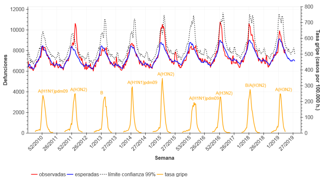
Figura 11. Mortalidad semanal por todas las causas e incidencia semanal de gripe. España. Hasta semana 13/2018.
