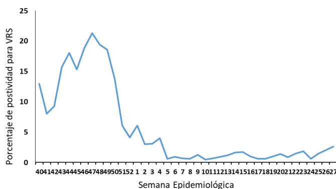
Figura 14. Porcentaje de positividad de VRS. Sistema no centinela. Temporada 2021-22. España
