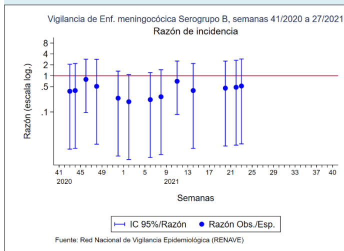
Figura 3. SEROGRUPO B
