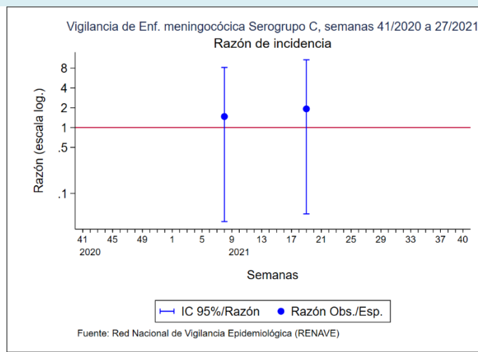
Figura 4. SEROGRUPO C
