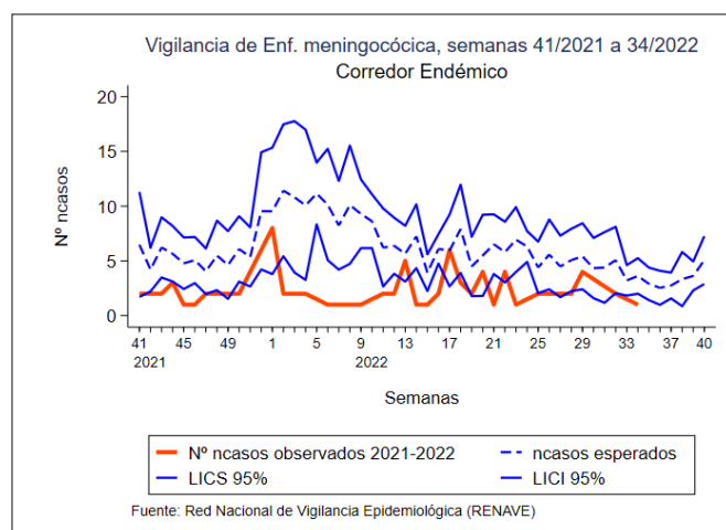
ENFERMEDAD MENINGOCÓCICA. [Semanas 41/2021 a 34/2022. Datos provisionales 4 ] Figura 1. Corredor endémico
