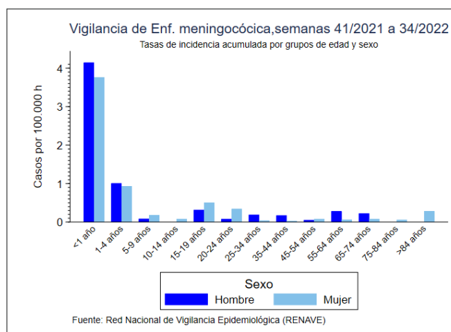
ENFERMEDAD MENINGOCÓCICA [Semanas 41/2021 a 34/2022. Datos provisionales 4 ] Figura 2. TI acumulada por grupo de edad y sexo
