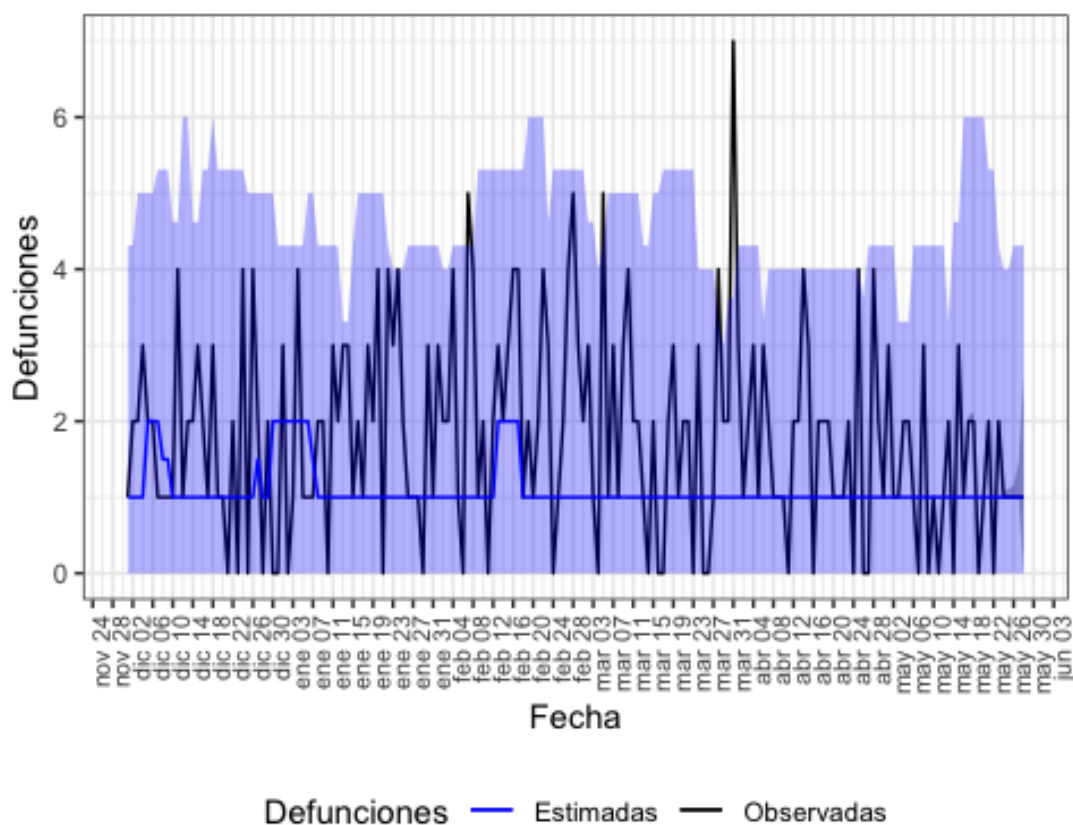
Figura 19. Mortalidad por todas las causas observada y esperada. Ceuta, diciembre 2019 hasta 28 de mayo de 2020.
