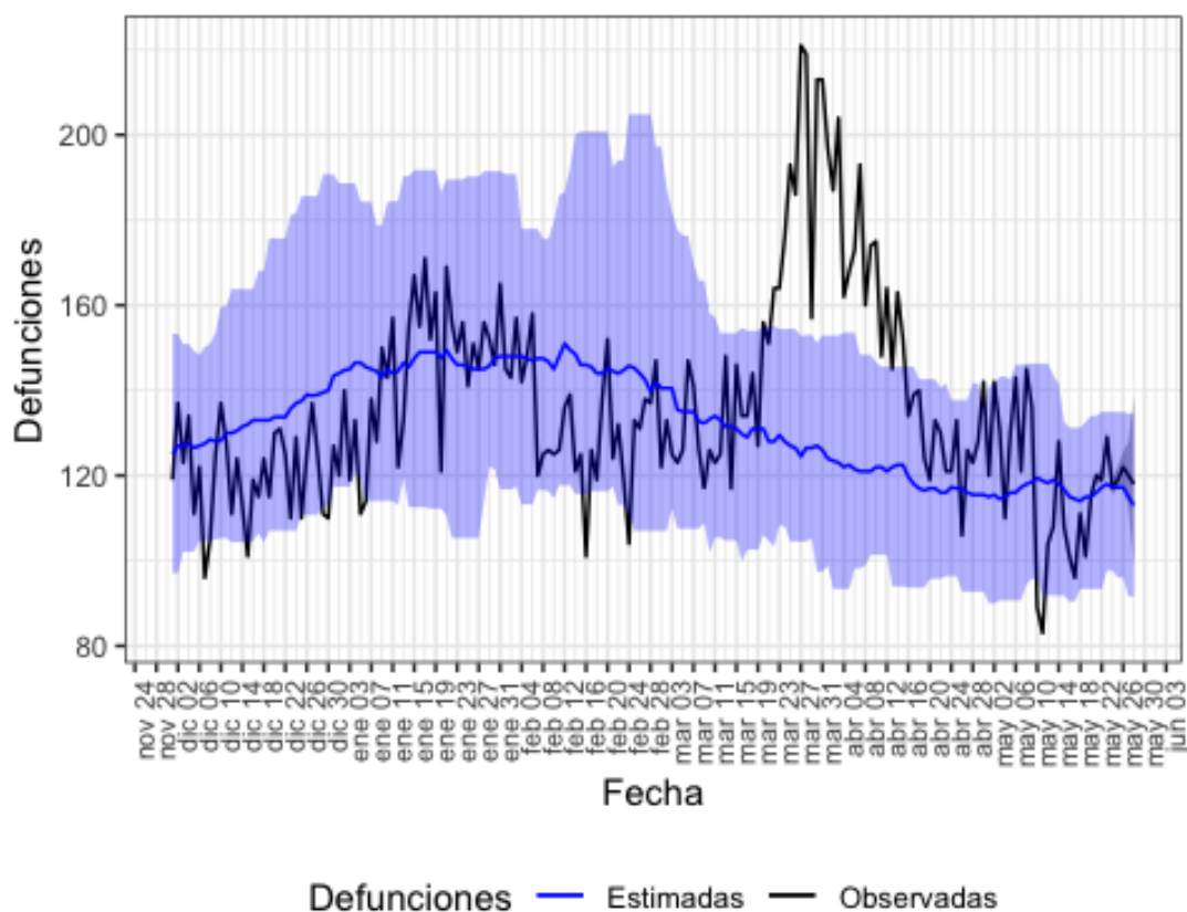
Figura 11. Mortalidad por todas las causas observada y esperada. Comunitat Valenciana, diciembre 2019 hasta 28 de mayo de 2020.
