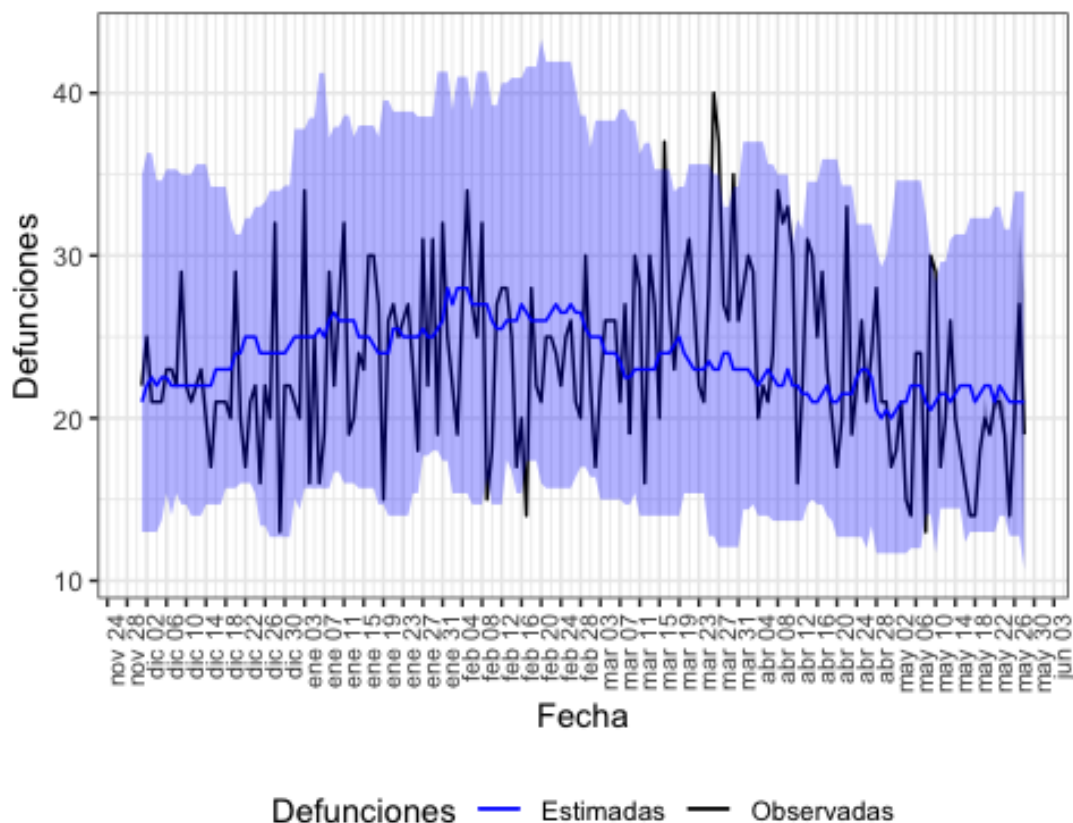
Figura 5. Mortalidad por todas las causas observada y esperada. Islas Baleares, diciembre 2019 hasta 28 de mayo de 2020.
