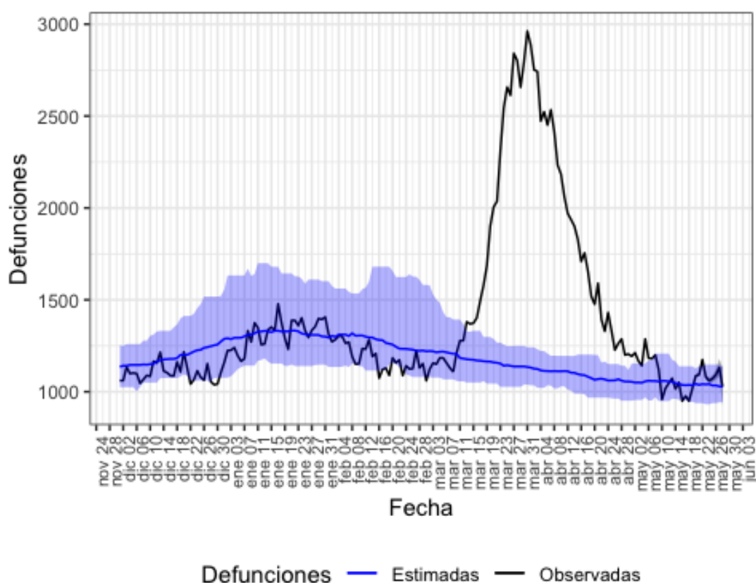
Figura 1. Mortalidad por todas las causas observada y esperada. España, diciembre 2019 hasta 28 de mayo de 2020
