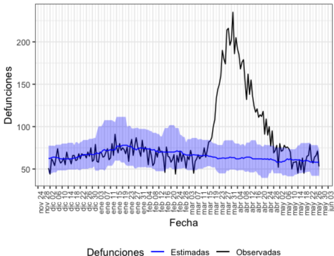
Figura 8. Mortalidad por todas las causas observada y esperada. Castilla y León, diciembre 2019 hasta 28 de mayo de 2020.
