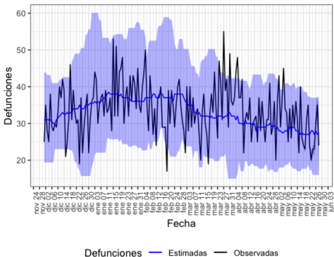
Figura 15. Mortalidad por todas las causas observada y esperada. Murcia, diciembre 2019 hasta 28 de mayo de 2020.
