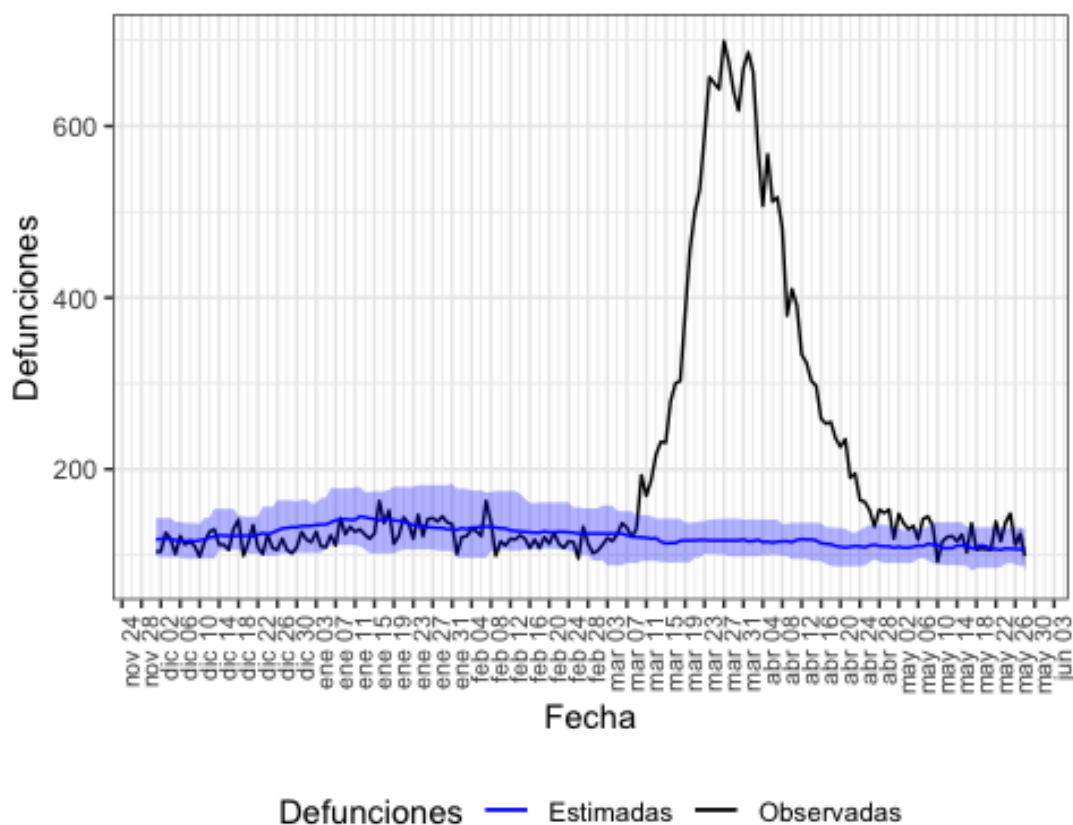
Figura 14. Mortalidad por todas las causas observada y esperada. Comunidad de Madrid, diciembre 2019 hasta 28 de mayo de 2020.
