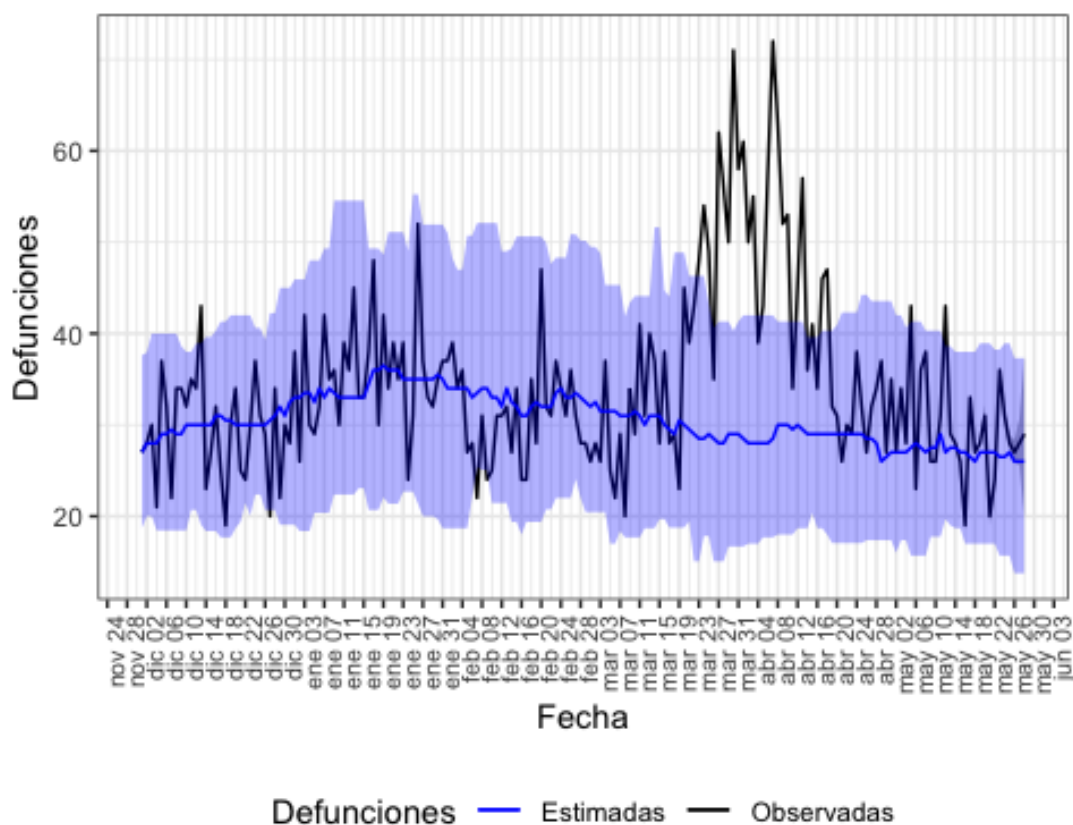
Figura 12. Mortalidad por todas las causas observada y esperada. Extremadura, diciembre 2019 hasta 28 de mayo de 2020.
