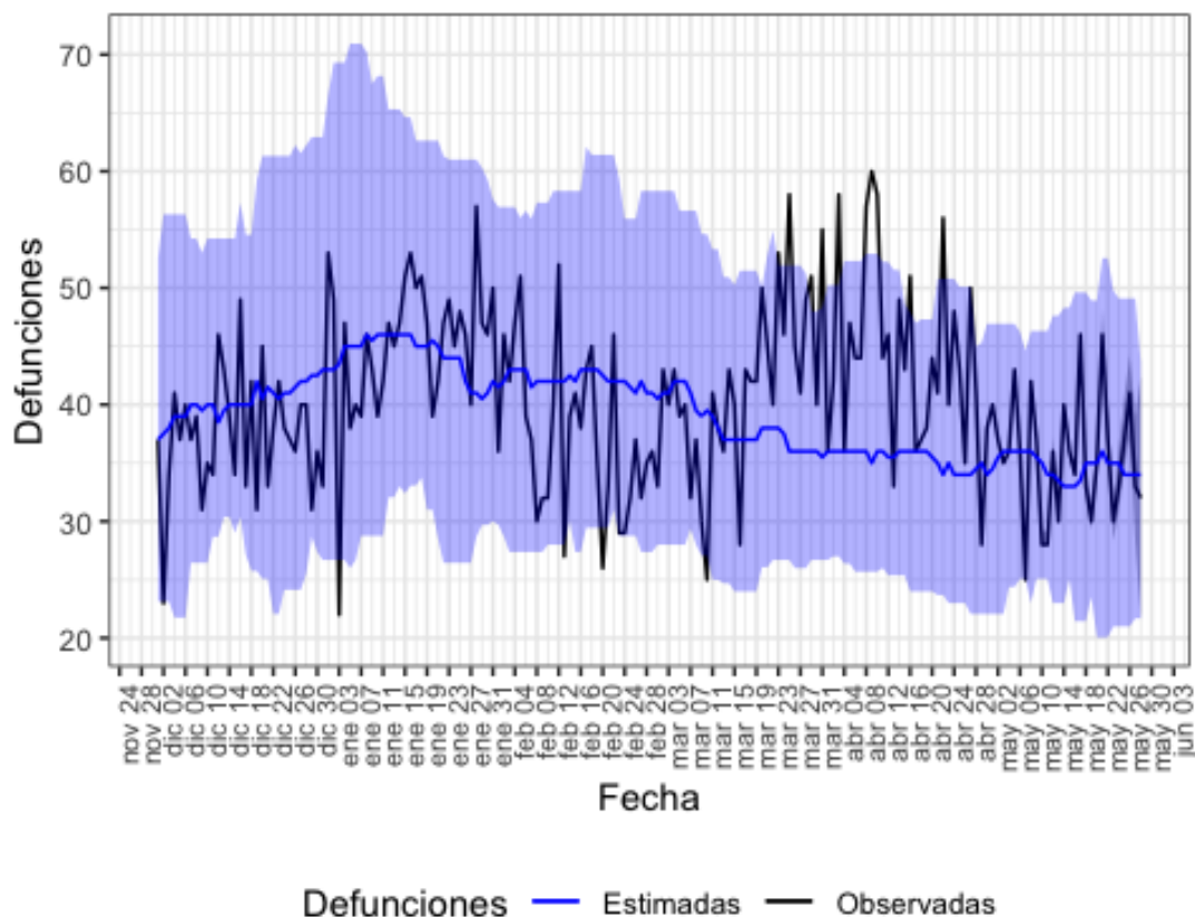
Figura 4. Mortalidad por todas las causas observada y esperada. Asturias, diciembre 2019 hasta 28 de mayo de 2020.
