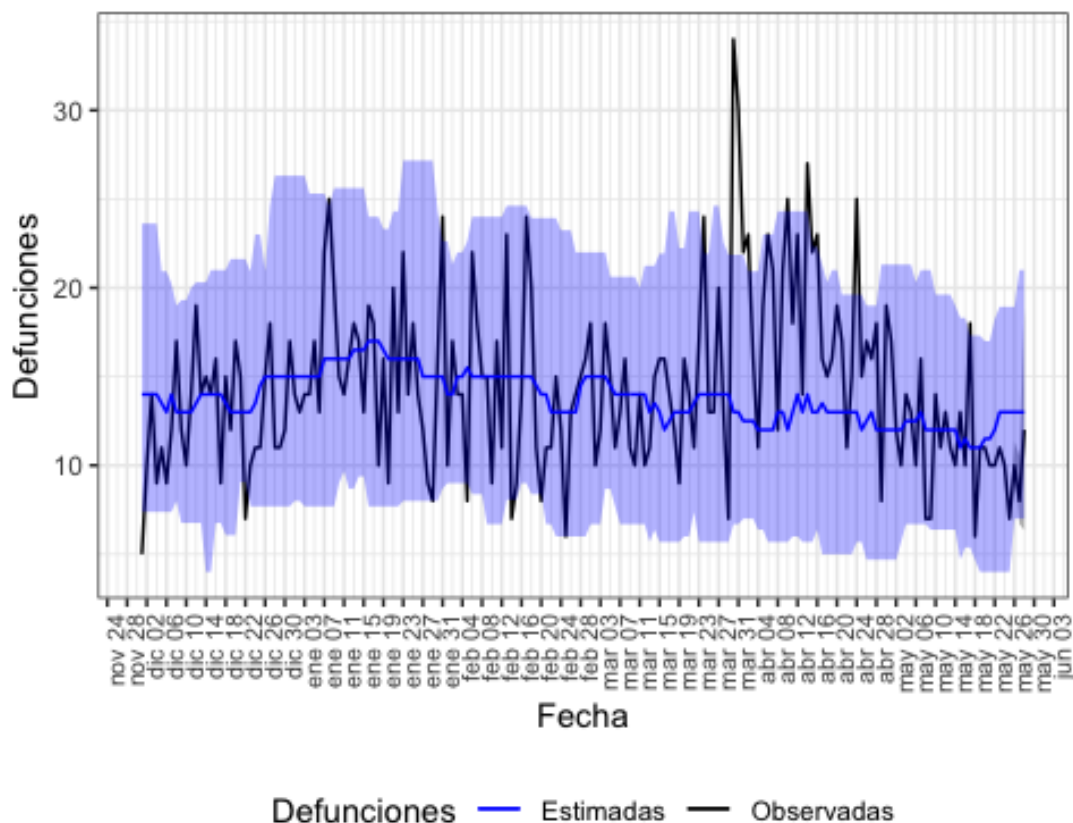
Figura 7. Mortalidad por todas las causas observada y esperada. Cantabria, diciembre 2019 hasta 28 de mayo de 2020.
