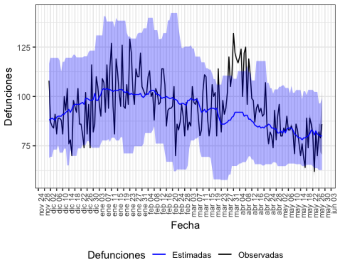
Figura 13. Mortalidad por todas las causas observada y esperada. Galicia, diciembre 2019 hasta 28 de mayo de 2020.
