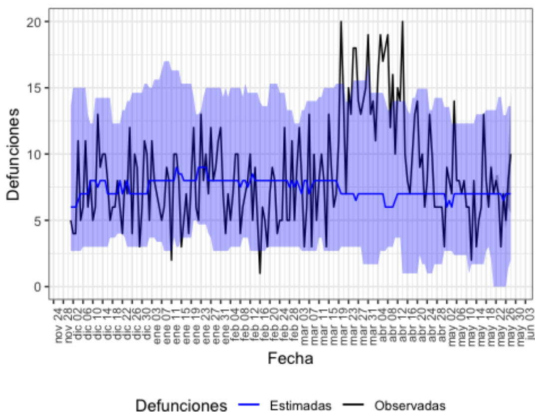
Figura 18. Mortalidad por todas las causas observada y esperada. La Rioja, diciembre 2019 hasta 28 de mayo de 2020.
