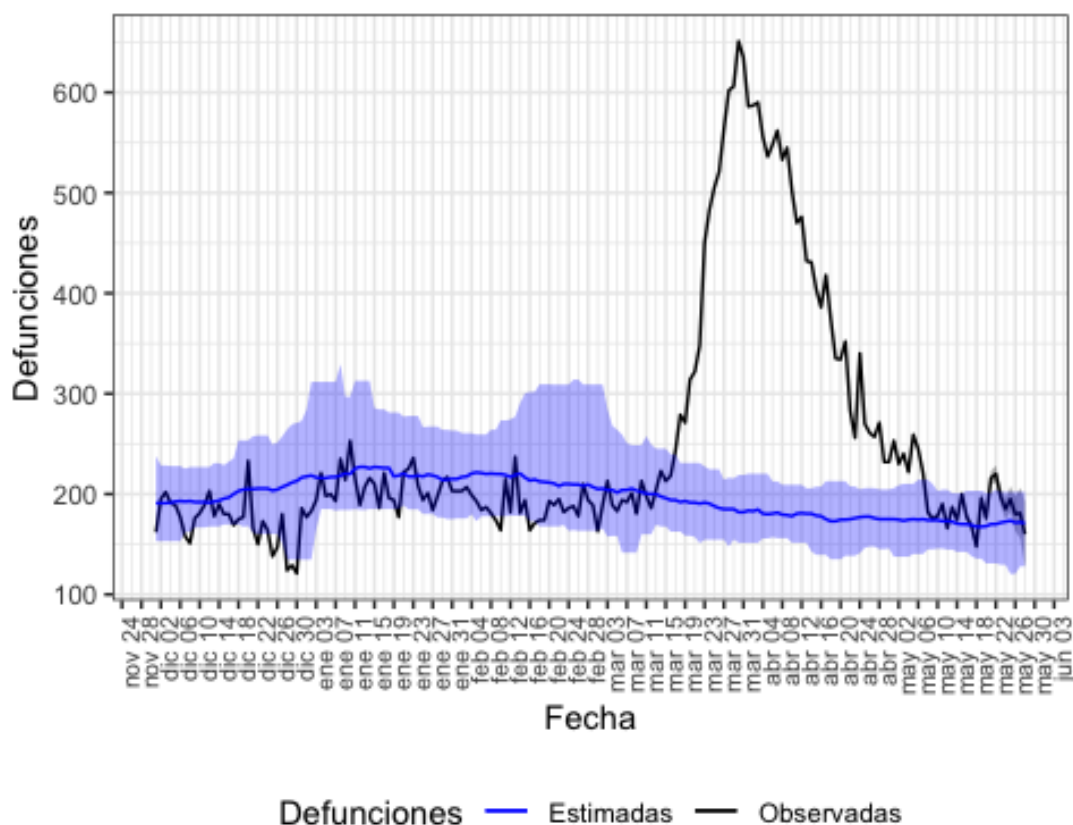
Figura 10. Mortalidad por todas las causas observada y esperada. Cataluña, diciembre 2019 hasta 28 de mayo de 2020.
