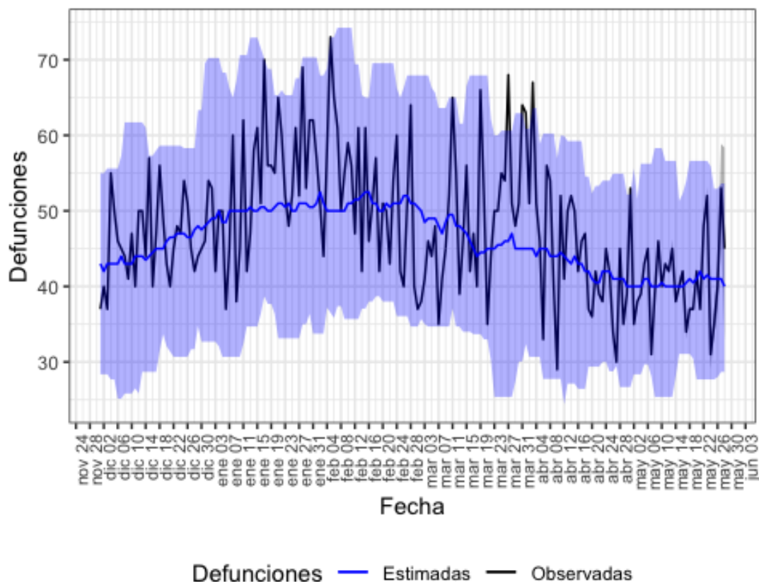
Figura 6. Mortalidad por todas las causas observada y esperada. Canarias, diciembre 2019 hasta 28 de mayo de 2020.
