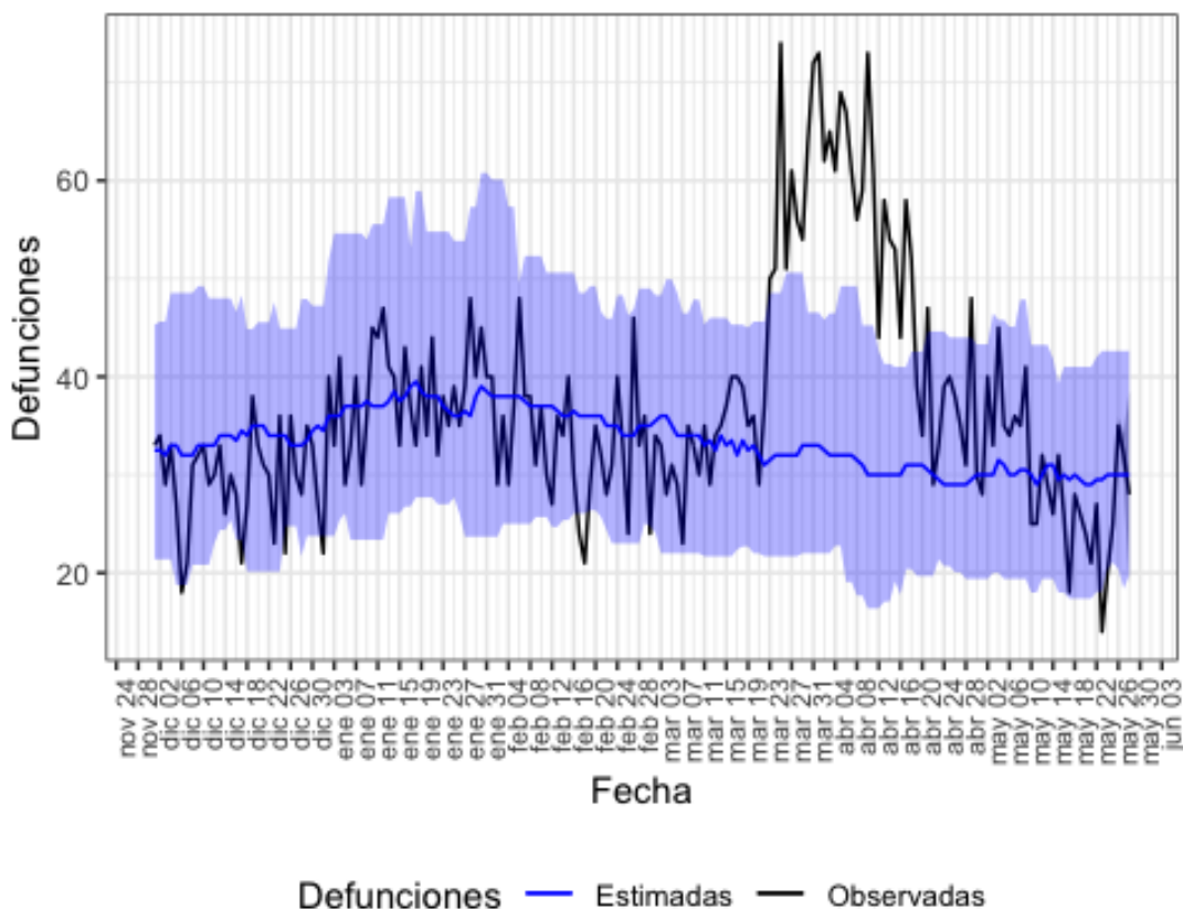
Figura 3. Mortalidad por todas las causas observada y esperada. Aragón, diciembre 2019 hasta 28 de mayo de 2020.
