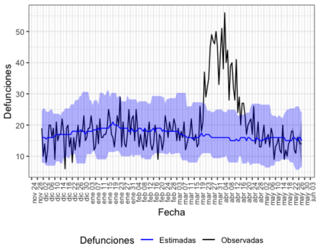
Figura 16. Mortalidad por todas las causas observada y esperada. Navarra, diciembre 2019 hasta 28 de mayo de 2020.
