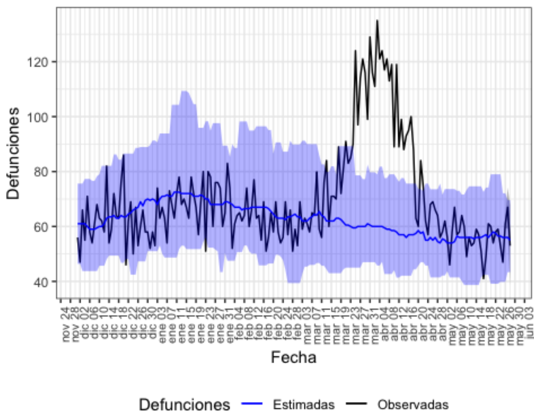
Figura 17. Mortalidad por todas las causas observada y esperada. País Vasco, diciembre 2019 hasta 28 de mayo de 2020.
