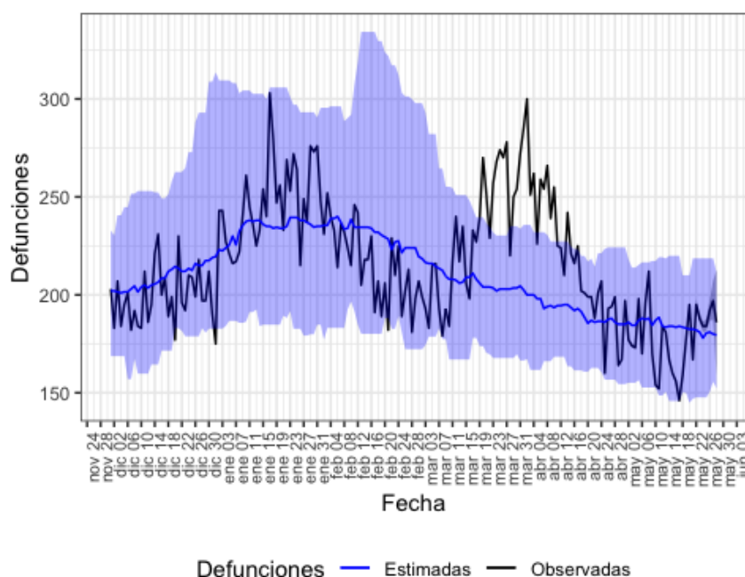
Figura 2. Mortalidad por todas las causas observada y esperada. Andalucía, diciembre 2019 hasta 28 de mayo de 2020.
